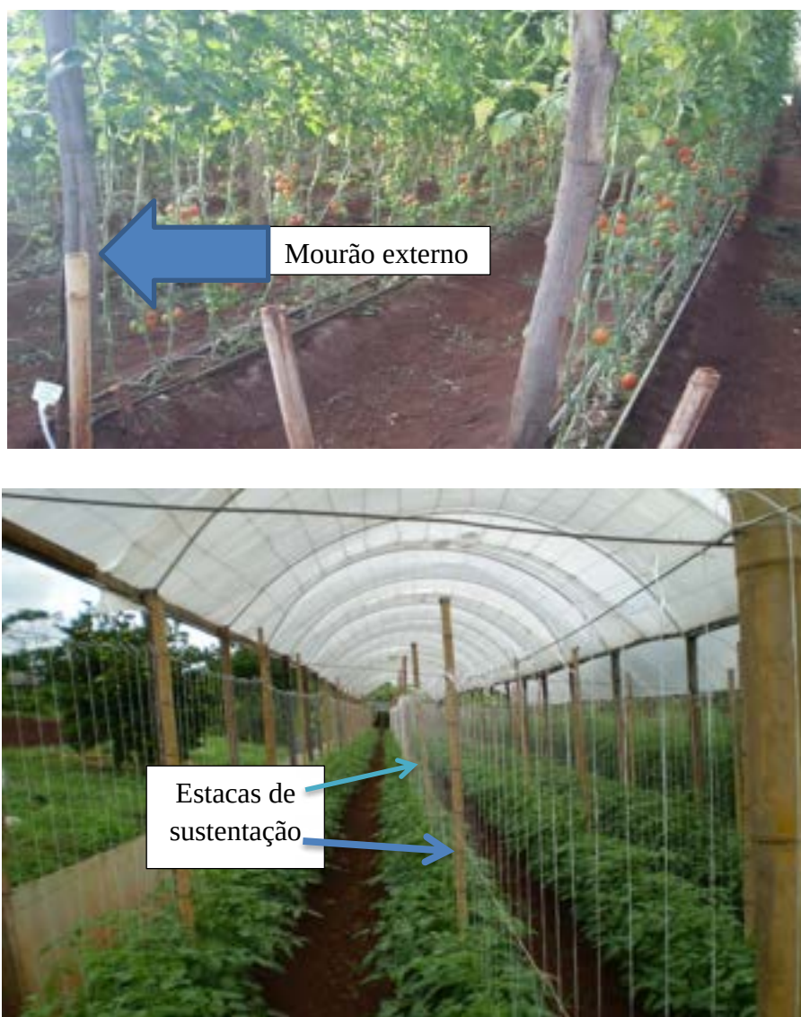
Figura 70. Estrutura de sustentação para condução vertical do Tomateiro
